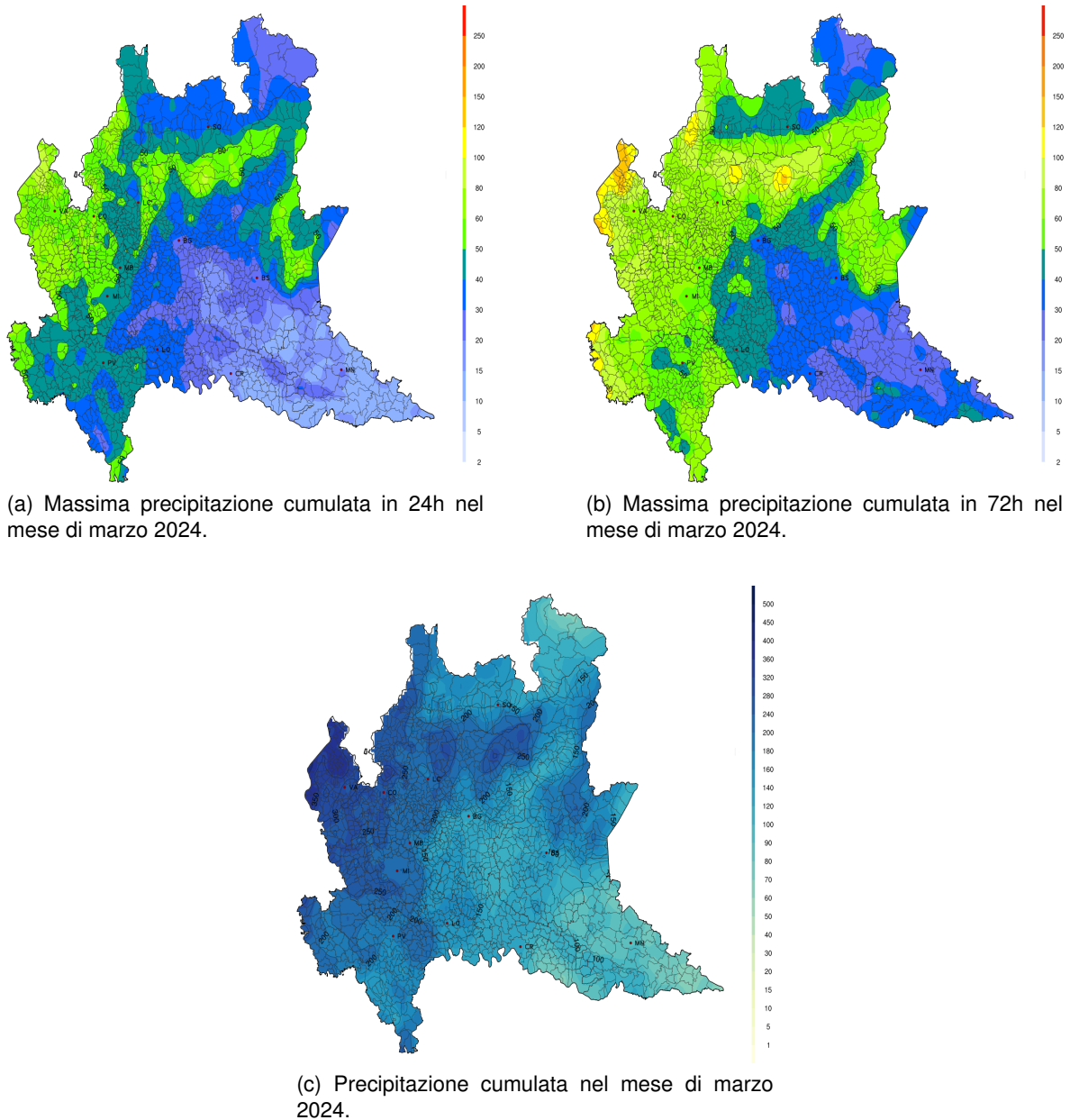
Figura 3. Valutazione del regime pluviometrico durante il mese di marzo 2024.
